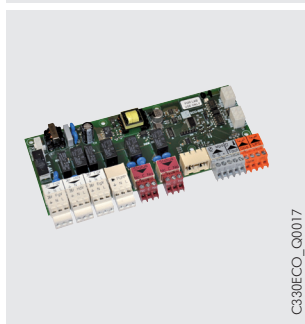
Плата SCU-S05 для подключения внешних устройств безопасности
