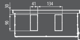
Вид с торца Ntherm 370.150 с U-образным бортом
