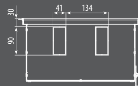
Вид с торца Ntherm 370.200 с F-образным бортом
