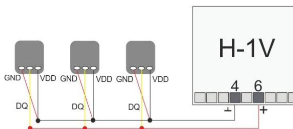
Датчик DS18B20
